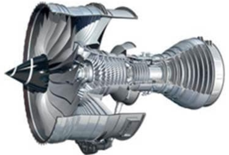
Trent XWB – A350 22 fan blades; 118 inch fan 97K Thrust
